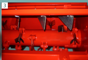
3 Τριπλά μαχαίρια & πτερύγια Triple knives & fins
