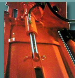
Υδραυλικό σύστημα μετατόπισης Hydraulic adjustment system
