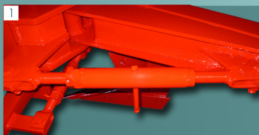
1 Ρύθμιση ανοίγματος με ραντάρ Width adjustment mechanical cylinder
