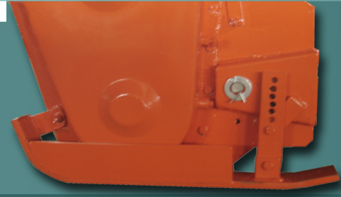
Πλευρική ρύθμιση βάθους Slides for depth regulation
