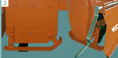
Μηχανική μετατόπιση & ρύθμιση βάθους Mech. adjustable offset & depth adjustment
