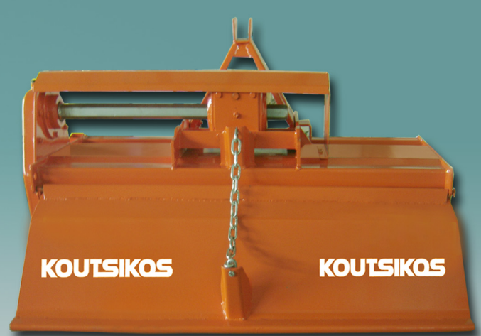
Πίσω όψη σταθερής φρέζας • Fix rotary tiller back view
