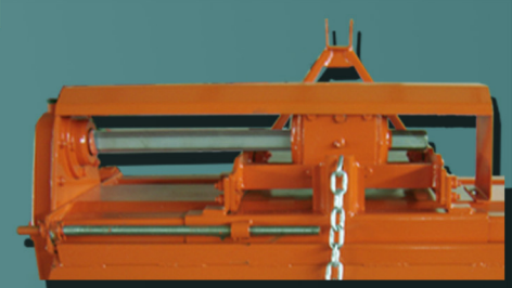
Πίσω όψη συρταρωτής φρέζας Adjustable offset back view
